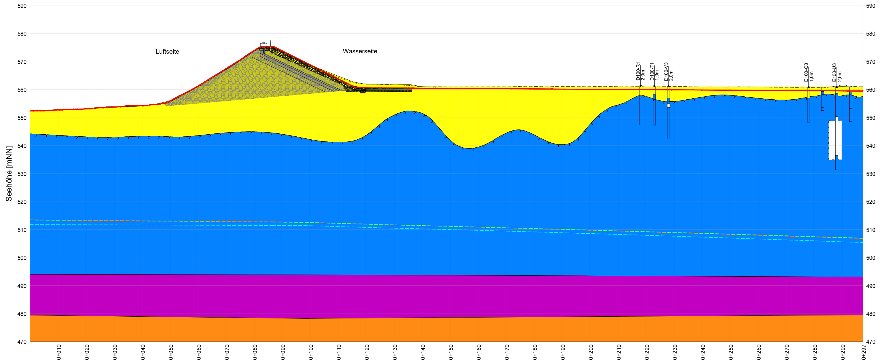
Geologischer Schnitt 0+360 Blickrichtung Nordosten M 1:400
