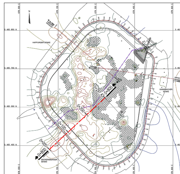
Übersicht Schnittführung Planausschnitt HAP-OB-020
