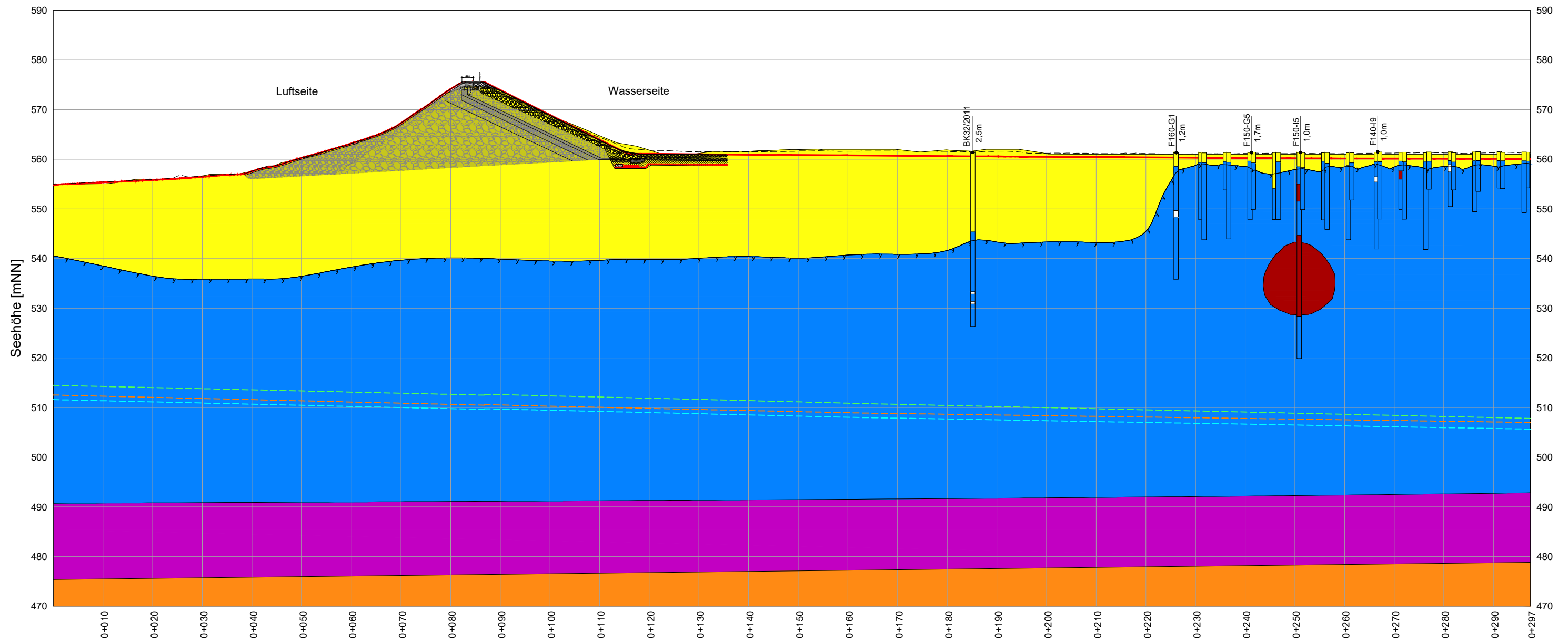
Geologischer Schnitt 0+800 Blickrichtung Nordwesten M 1:400
